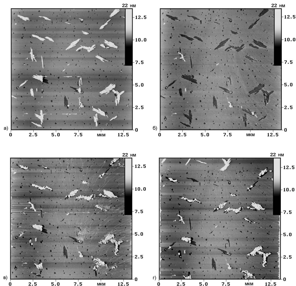
Рис. 5.3. Кристаллиты в монослое бегеновой кислоты, осажденной на подложку слюды методом ГО с поверхности субфазы, содержащей CdTe кластеры (динамика разрушения/восстановления).
